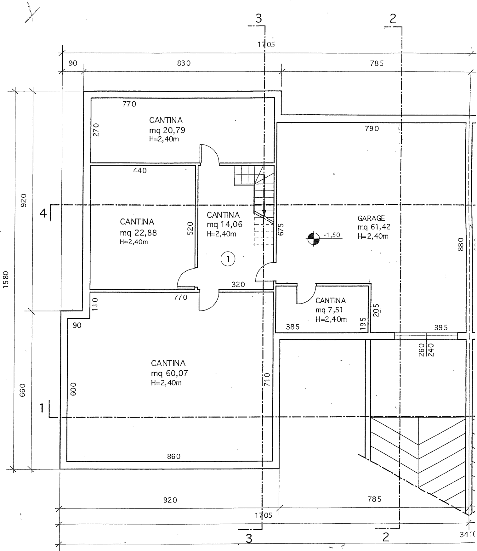
PIANTA PIANCO scala
