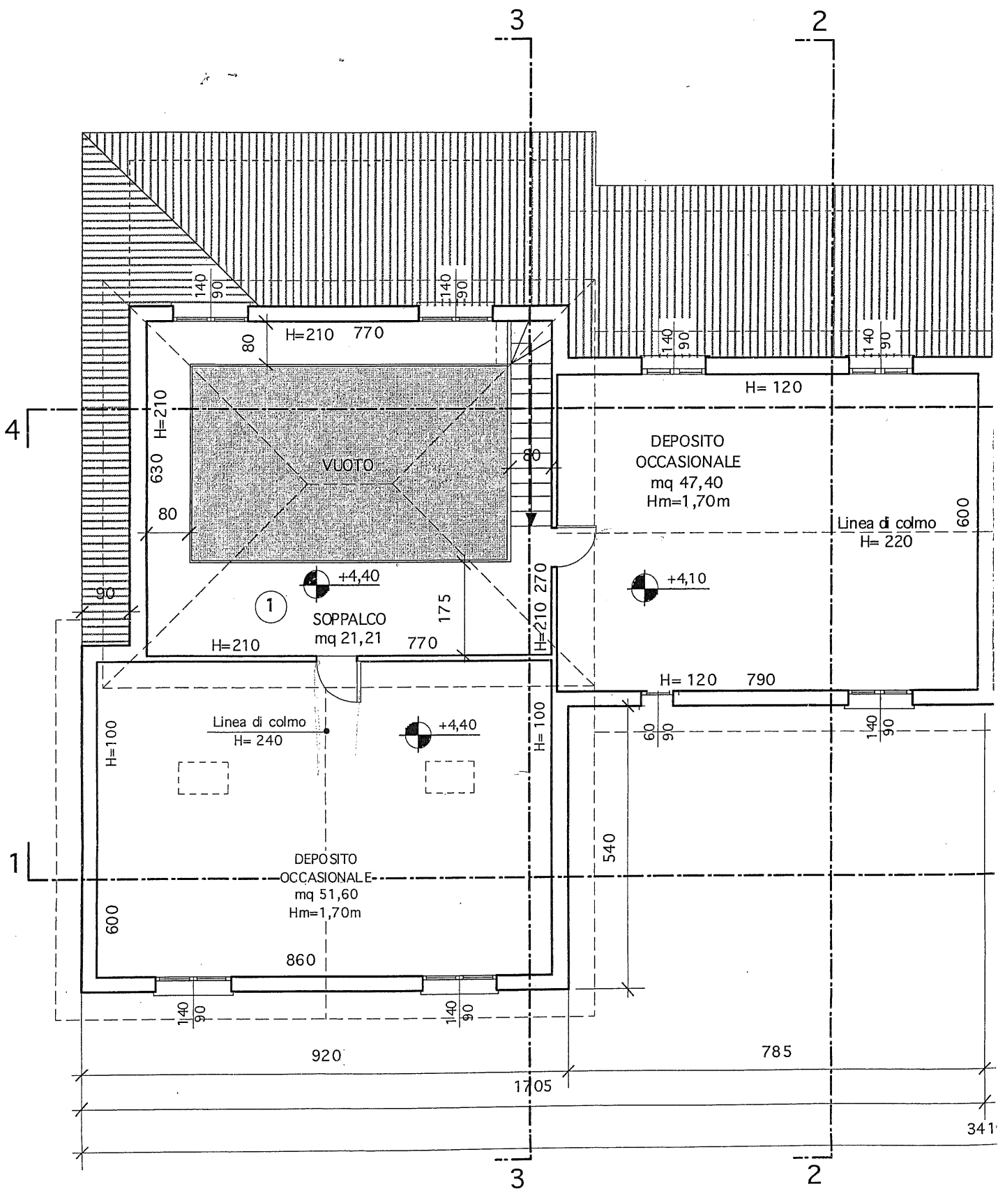
PIANTA PIANO scala 1
