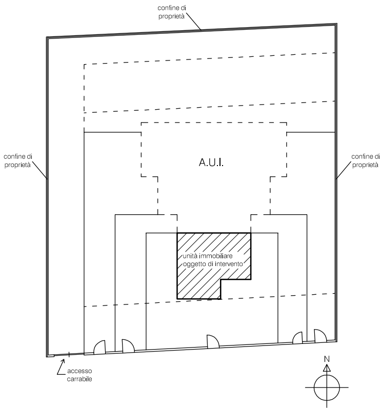
PLANIMETRIA 1:200
