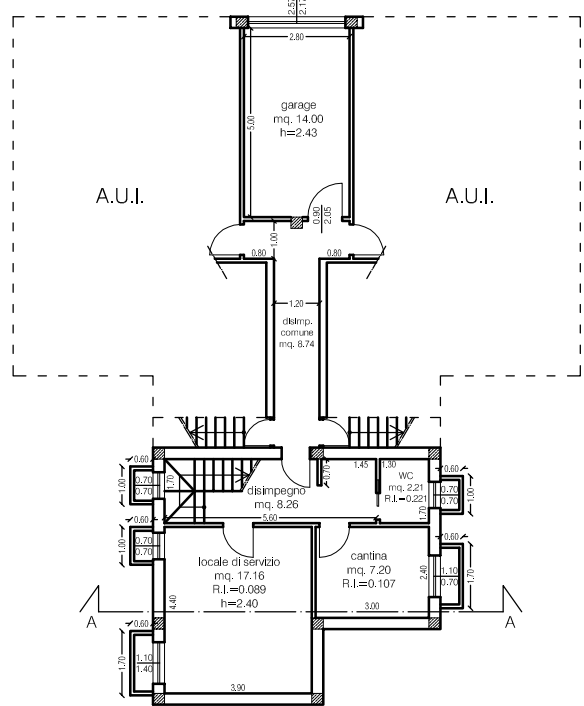
PIANTA PIANO SEMINTERRATO
