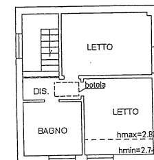
PIANO PRIMO H=2.80
