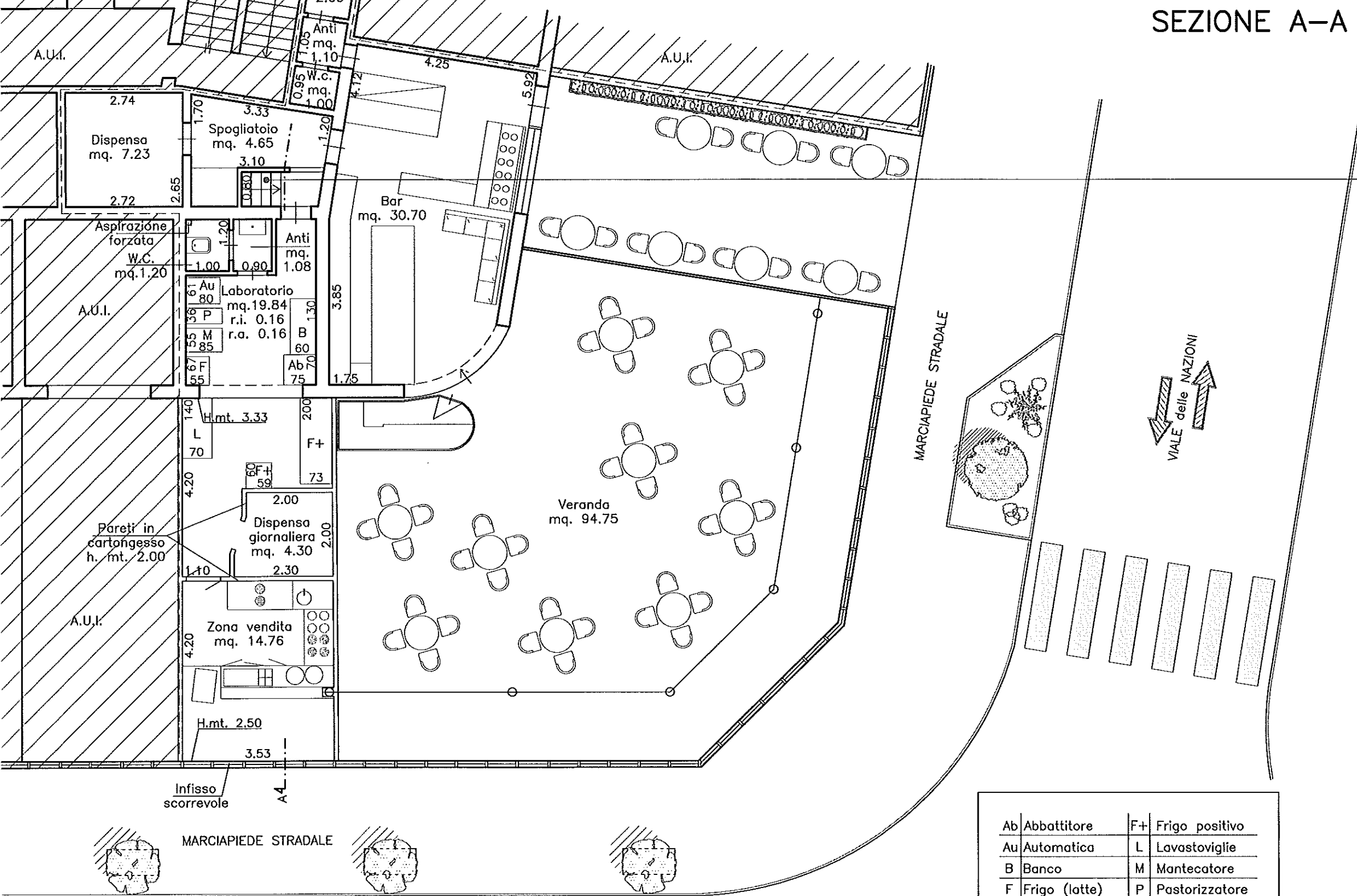
LEGENDA MACCHINARI
